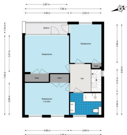
Oud Over 48 - Loenen aan de Vecht Tweede verdieping
